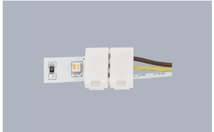
Verdrahteter Steckverbinder für CX STRIP
